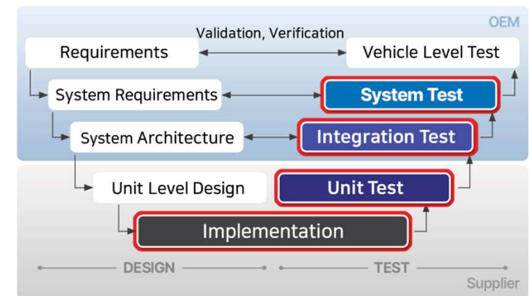
차량 개발 프로세스 - 통신 검증
